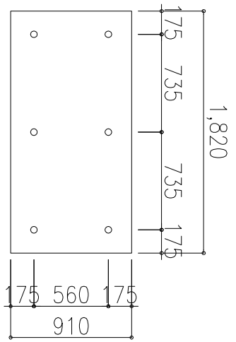
図中使用パネル詳細 S=1/1 UP250TE4
