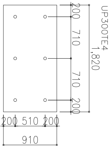
図中使用パネル詳細図 S=1/1
